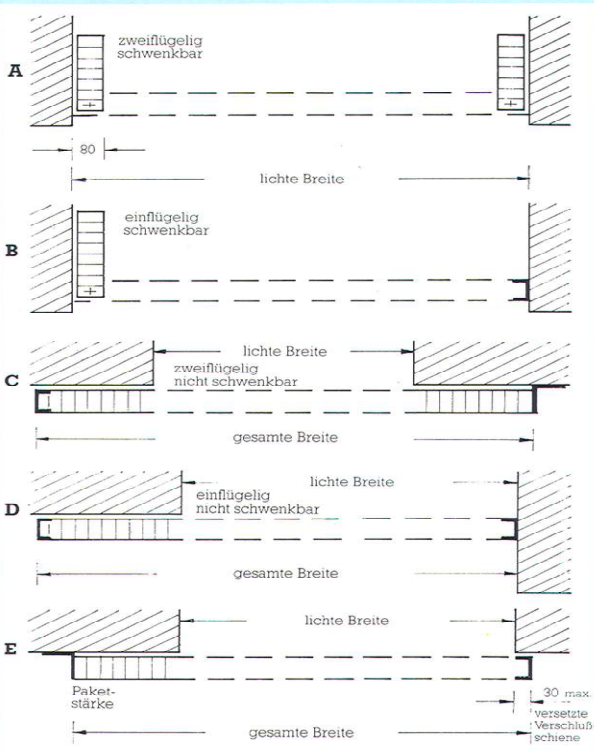
Grundriß-Anordnungen
