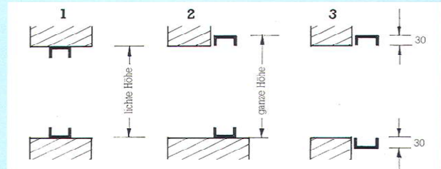
Höhenschnitte
