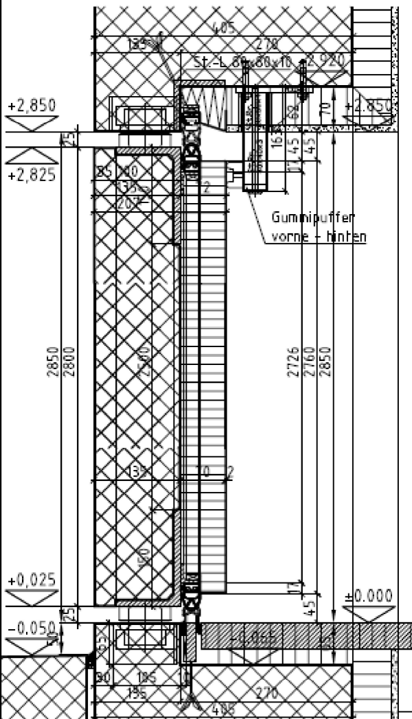
Vertikalschnitt Mst: 1:5
