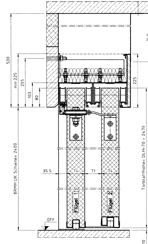
Schnitt B-B
